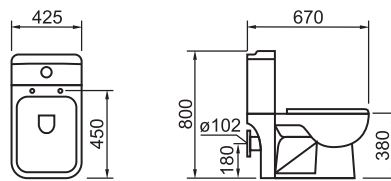
UC11011P Monoblok baltik - komplet Priključak vode sa donje leve strane
